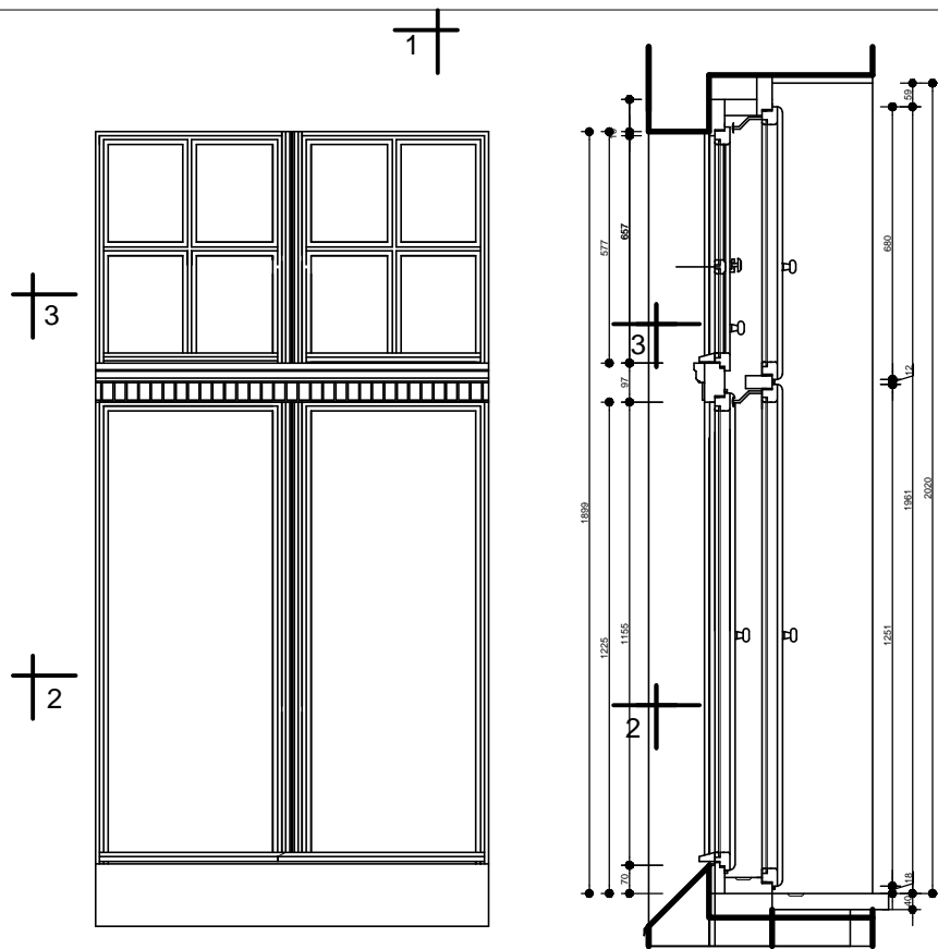
WYKONANIE OKNA I DRZWI SKALA 1:10
