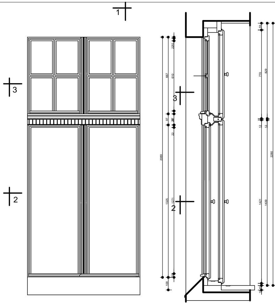
WYKONANIE OKNA SKALA 1:10
